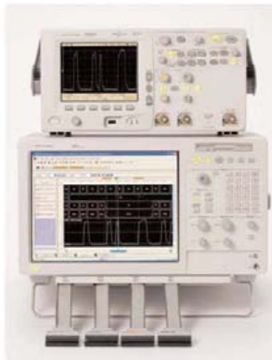
Рисунок 9 - Выполнение коррелированных по времени измерений между логическим анализатором компании Agilent и осциллографом серии 6000
